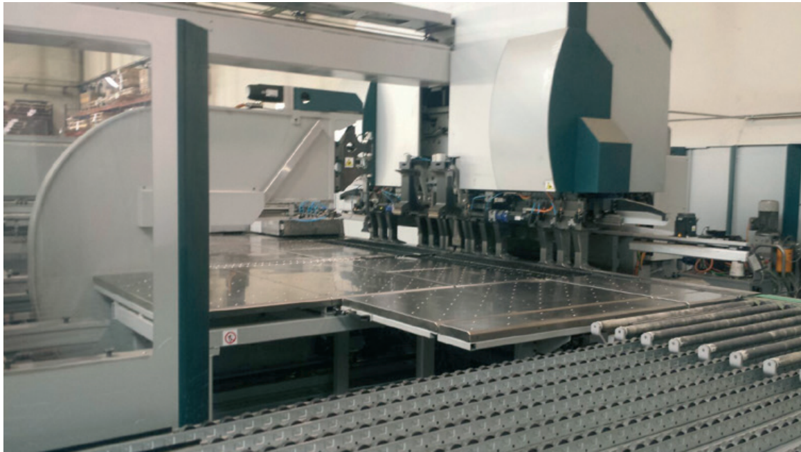
La paneladora es capaz de plegar piezas de hasta 2200 mm de largo por 250 mm de altura, con espesores de 3,2 mm, habituales para Salvagnini
